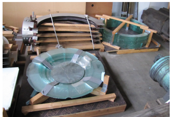
Teile der Glaskugel und Stahlbügel
